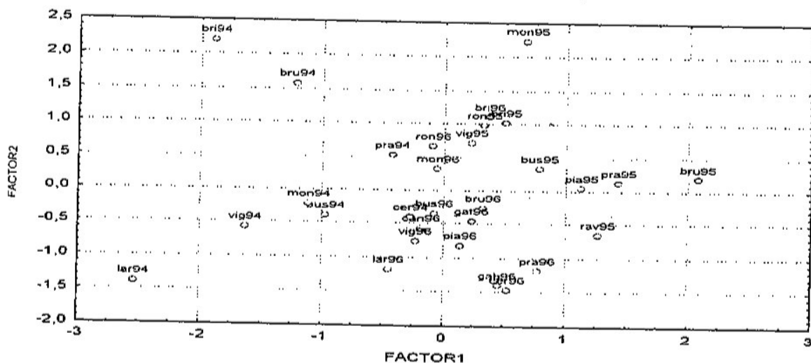
Fig. 5 - Distribution avec données standardisés des variables enologiques de la figure précédente.
