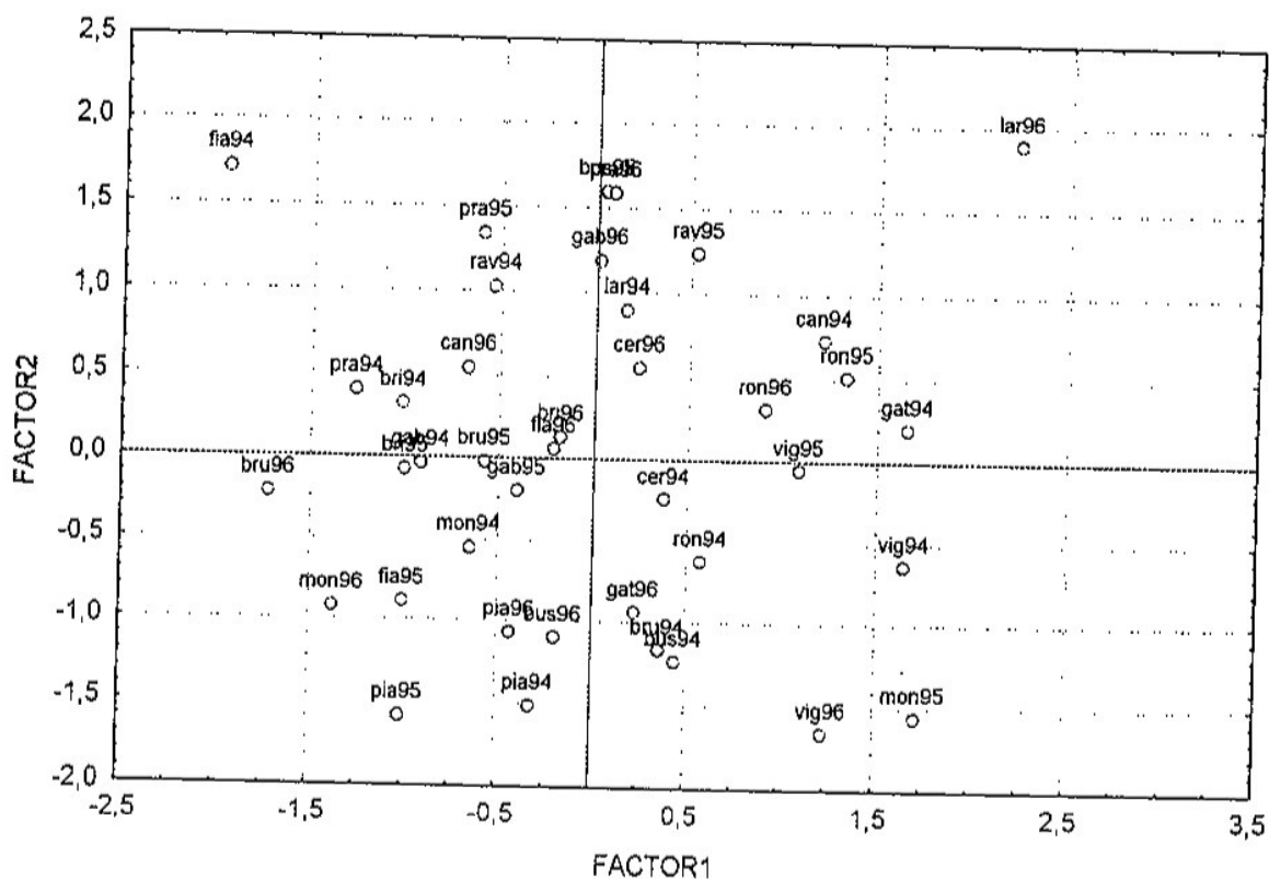
Fig. 5 - Distribution avec données standardisés des variables enologiques de la figure précédente.
