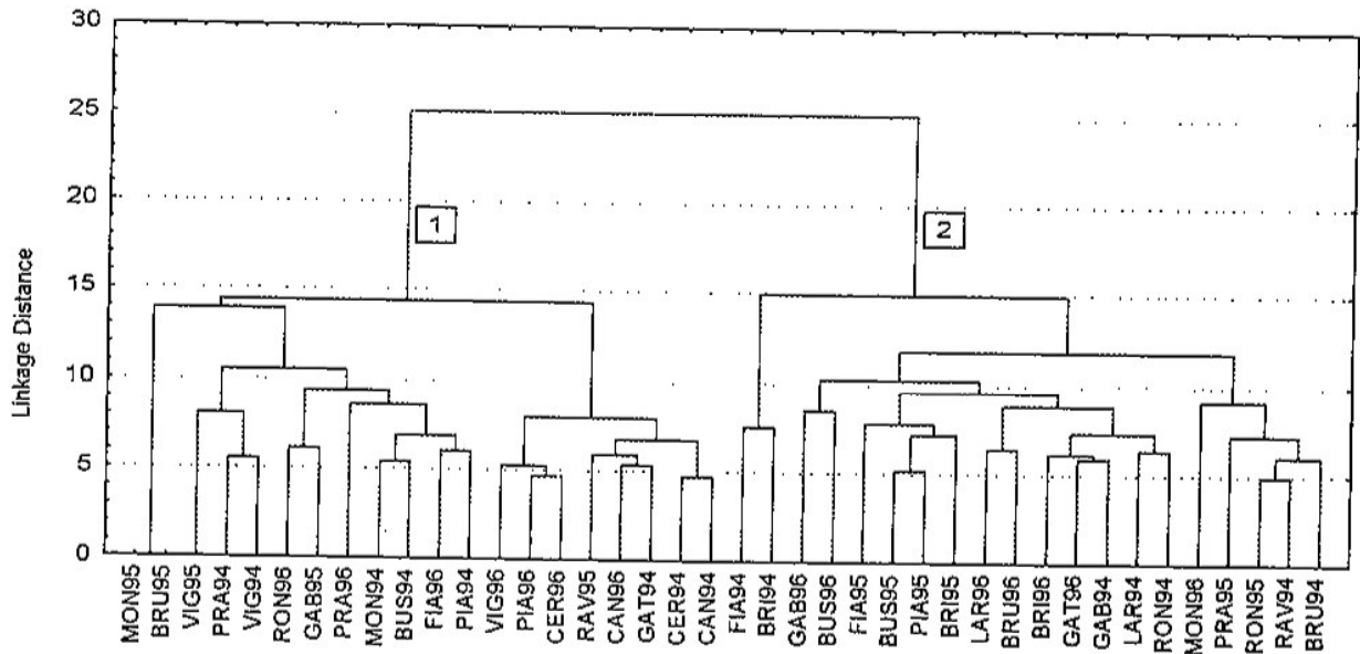
Fig.3 - Clusters analysis sur valeurs standardisés de l'analyse sensorielle des vins.
