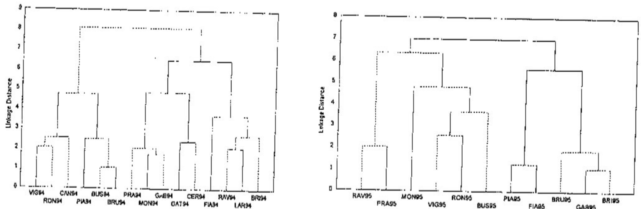
Fig. 7 - Clusters analysis. Moûts 1994, 1995 (dessus) et 1996 (dessous). Pour ce dernier on peut voir 2 groupes (A e B). Les différences principales sont causées par sucres, anthocyanes, flavonoides totales, acidité.
