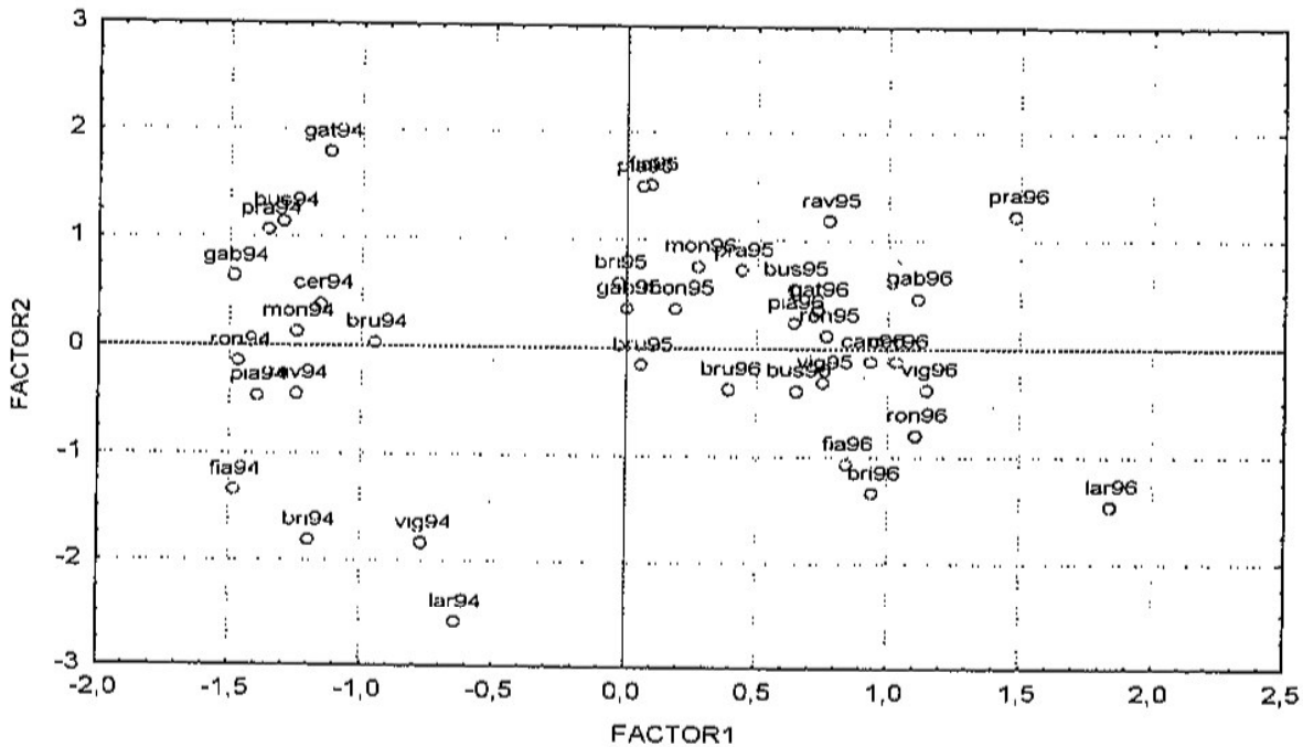
Fig. 4 - Distribution sur le plan obtenu par les deux composantes principales des moûts et des grappes des trois ans d'expérimentation. En évidence l'effet millésime, surtout pour le 1994. Les variables utilisées sont: anthocyanes et flavonoïdes des peaux des baies, sucres, acide citrique, malique et tartrique, acidité totale du moût. La variation expliquée par les deux composantes c'est 76.2 %.
