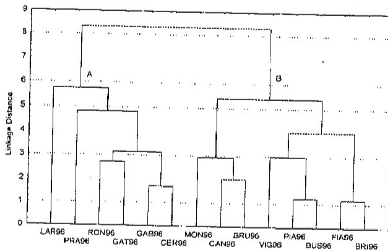
Fig. 7 - Clusters analysis. Moûts 1994, 1995 (dessus) et 1996 (dessous). Pour ce dernier on peut voir 2 groupes (A e B). Les différences principales sont causées par sucres, anthocyanes, flavonoides totales, acidité.
